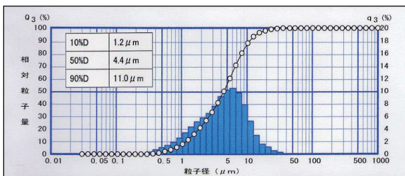
粒度分布図例
