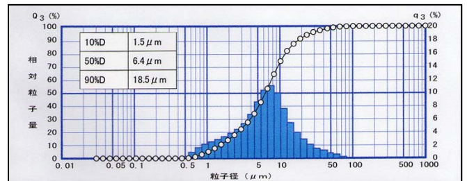
《MODEL. NO750》粒度分布図例
