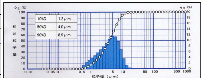
《MODEL. NO1500》粒度分布図例
